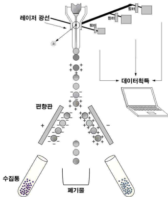
<그림 1> 유세포 분석기 기본 구조도
